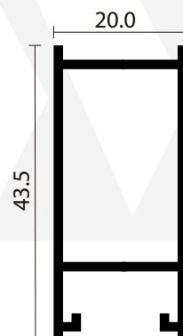
ALNA388 TRASLAPE
