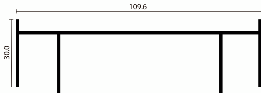
ALN700 CABEZAL
