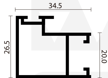
ALN391 ENGANCHE
