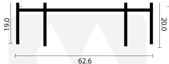
ALN392 CABEZAL DOS RIELES
