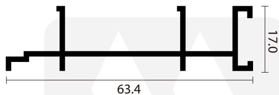
ALN387 SILLAR DOS RIELES
