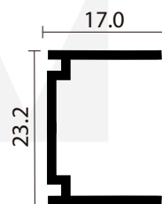
ALN403 ADAPTADOR
