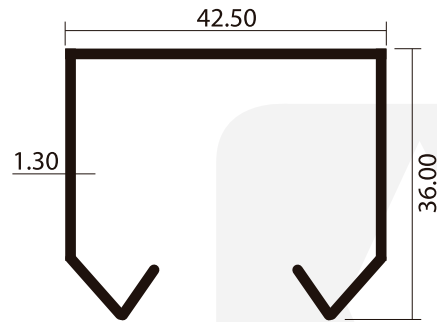
S391 Riel closet
