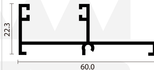
ALNA388 TRASLAPE
